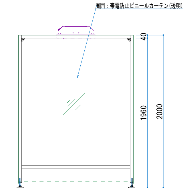
A矢视图
